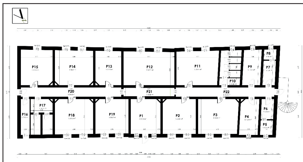
Obr. 8. Panský dom Wertheimstein - prízemne zameranie
