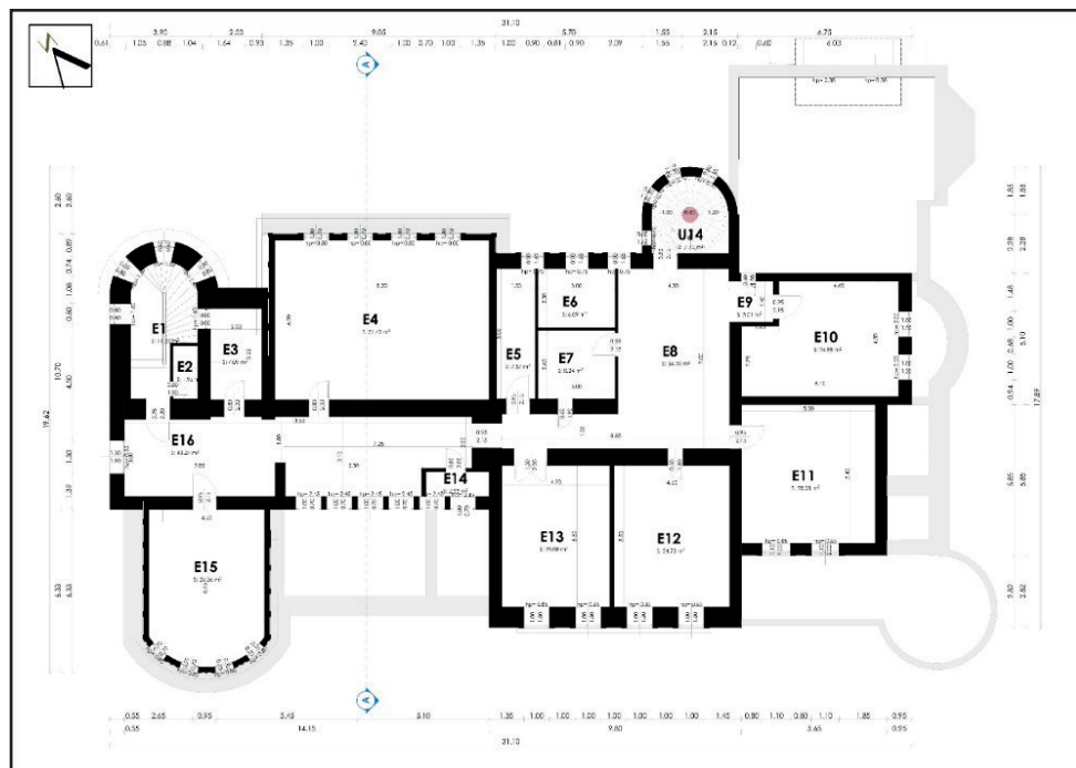
Obr. 14. Zámok Wertheimstein-Rothschild, poschodové zameranie
